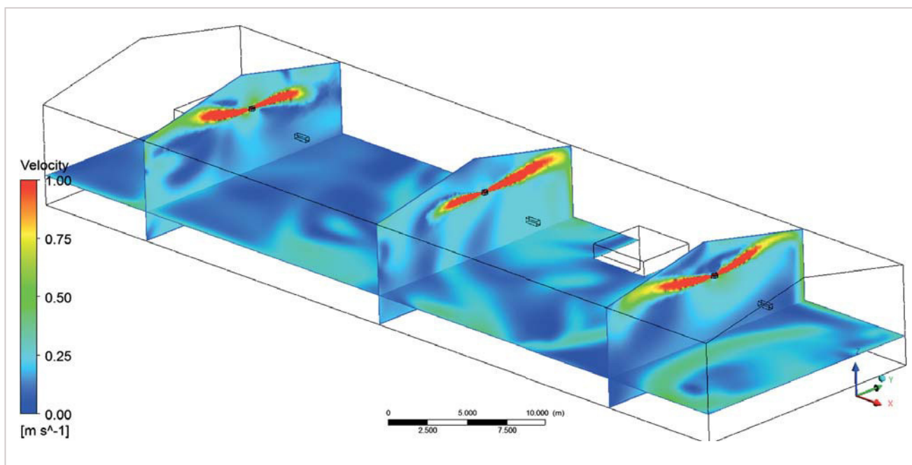
Рис. 5. Поля скоростей в объеме цеха при подаче воздуха через диффузоры ДИН 400
